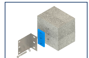
Abb. 1.2 Verbindungen zwischen Mauerwerk- und Verschalung
