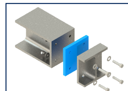
Abb. 1.1 Stahl-Stahl-Verbindung zwischen Innen- und Außenelementen
