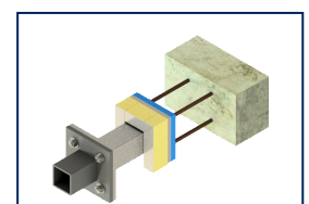
Abb. 1.4 Stahl-Beton-Verbindungen
