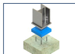
Abb. 1.3 Sockelverbindung
