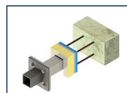
Abb. 1.4 Stahl-Beton-Verbindungen
