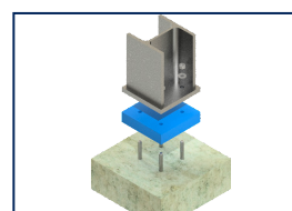
Abb. 1.3 Sockelverbindung
